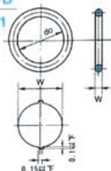
O 形圈尺寸
